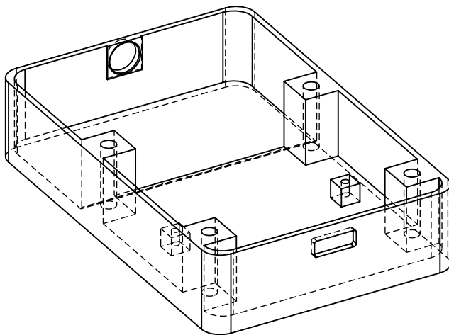
Vue isométrique à l'échelle 1:1
